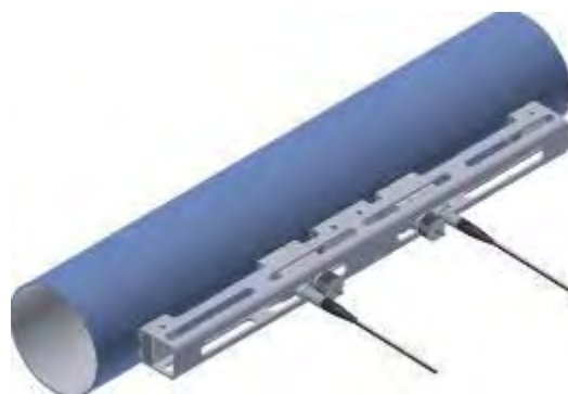
Рисунок 22. Накладной УЗП SE 1815 Пример установки на трубопроводе
